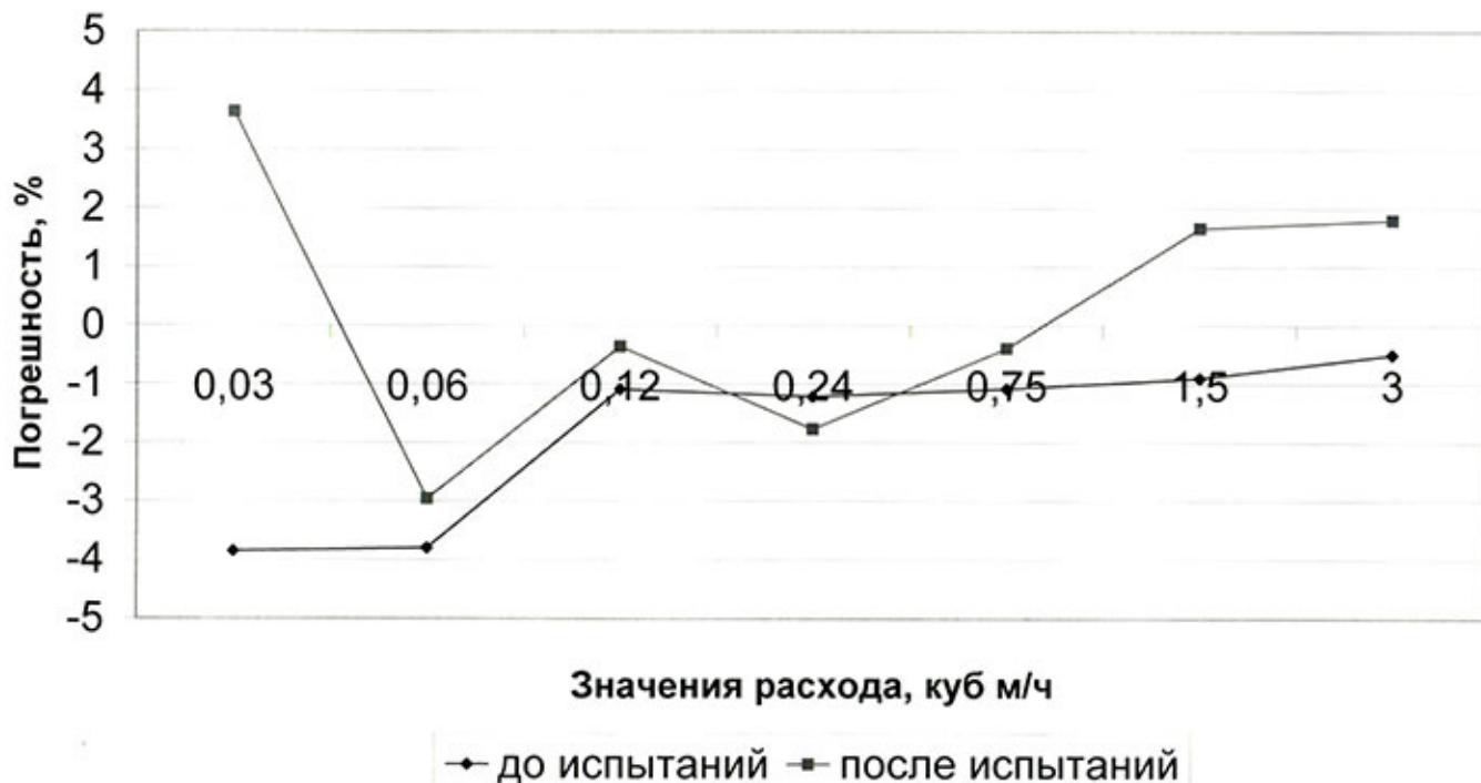
Сравнение характеристик счетчиков воды типа БЕРЕГУН до и после испытаний на ускоренный износ № 07 110061
